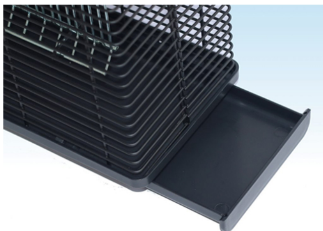
Vệ sinh khay hứng muỗi: Tắt đèn, rút nguồn trước khi vệ sinh. Tháo khay bằng cách rút ra ( với đèn CN16 | CN30), hoặc mở lẫy (với đèn CN100 Pro | CN150 Pro) như hình.
